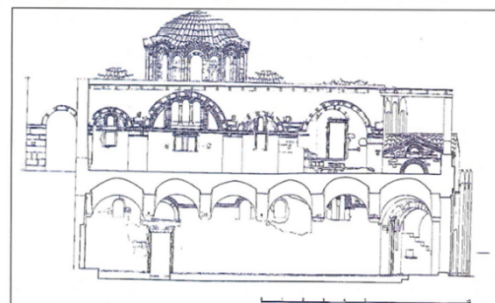
Τομή του ναού
