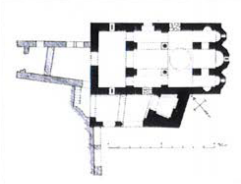
Κάτοψη του ναού
