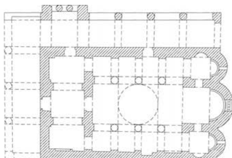
Κάτοψη ισογείου με το ιερό και τα τρία κλίτη
